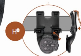
8K25 PASADOR CINTURÓN BELT LOOP PASSANT DE CEINTURE En polímero estampado Con sistema de apertura mediante pasadores con bloqueo Sistema giratorio 90° a la izquierda o a la derecha.
